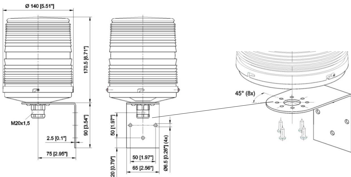
Abbildung 6 – Winkelmontage
