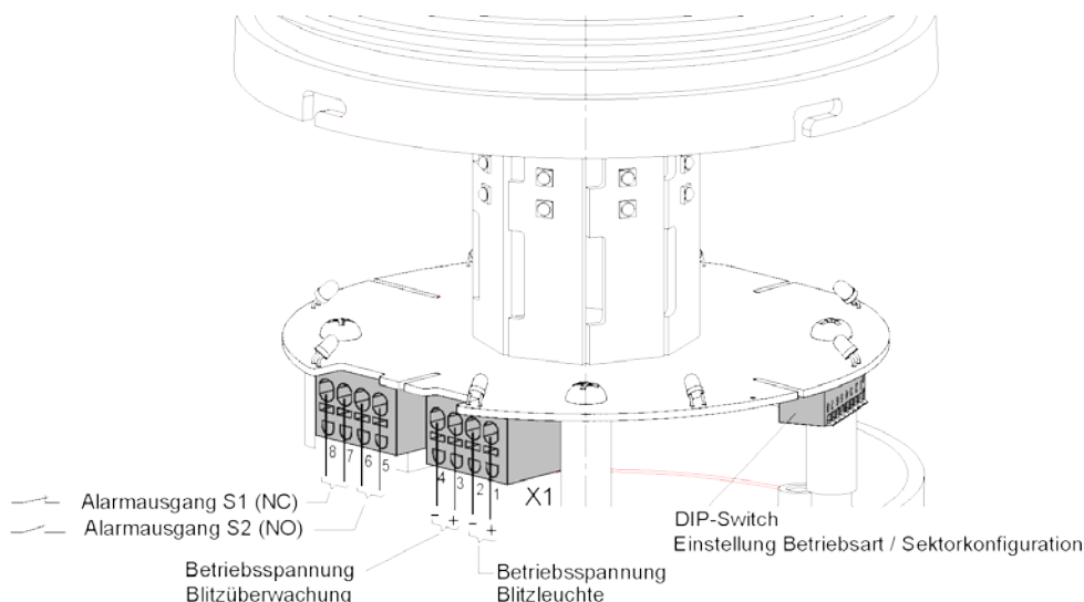
Abbildung 8 - Klemmenbelegung
