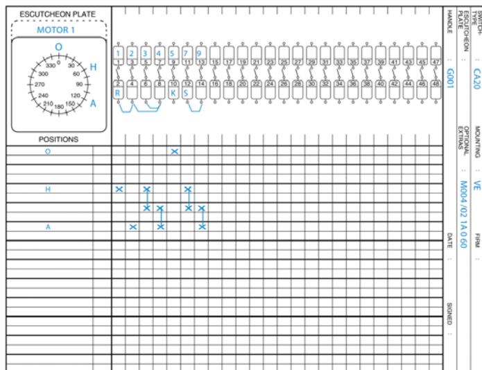
Przykładowa tabela programu łączeń
